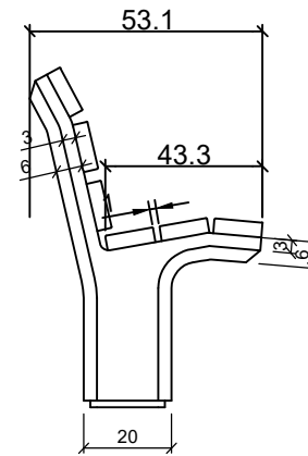
PERFIL / PROFILE
