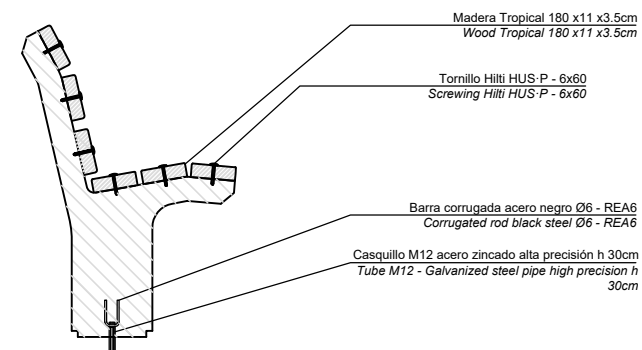
SECCION / SECTION
