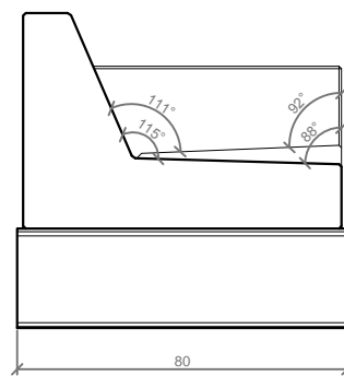
SECCIÓN A-A' / SECTION A-A'
