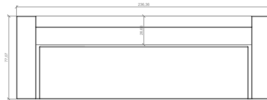
PLANTA / TOP VIEW
