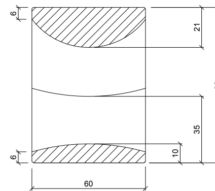
SECCIÓN A-A' / SECTION A-A'
