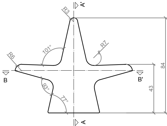
PERFIL / PROFILE
