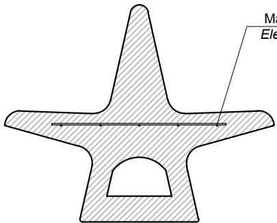
SECCION / SECTION
