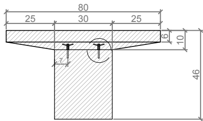
SECCION A-A' / SECTION A-A'
