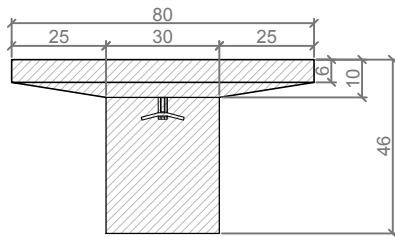
SECCION B-B' / SECTION B-B'
