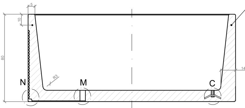
SECCION A-A' / SECTION A-A'
