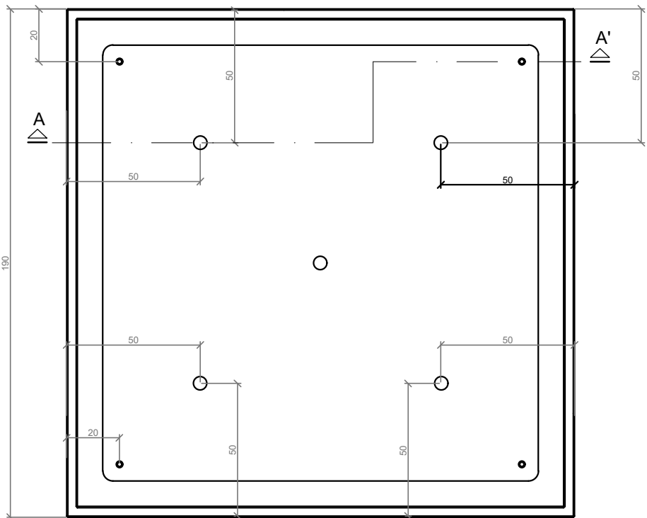
PLANTA / TOP VIEW
