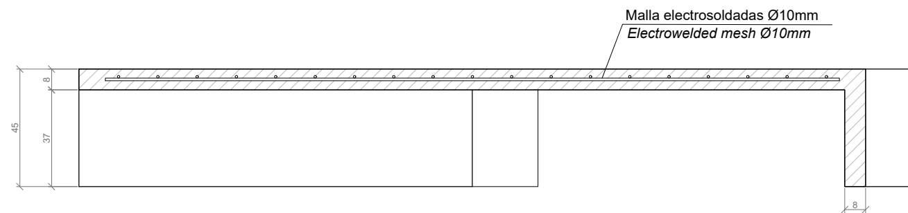
SECCIÓN / SECTION
