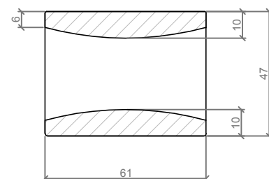
SECCION A-A' / SECTION A-A'
