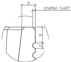
DETALLE C-C' / DETALLE C-C'
