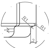
DETALLE B-B' / DETAIL B-B'
