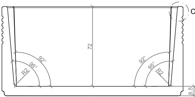
SECCION A-A' / SECTION A-A'
