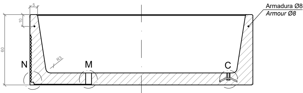
SECCION A-A' / SECTION A-A'
