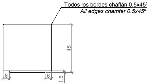
PERFIL / PROFILE
