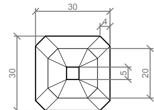
PLANTA / TOP VIEW
