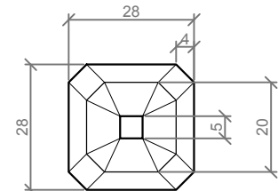
PLANTA / TOP VIEW
