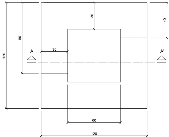
PLANTA / TOP VIEW
