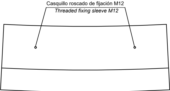
PLANTA INFERIOR / BOTTOM VIEW
