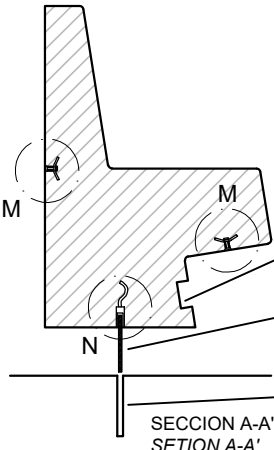
SECCION A-A' SECTION A-A'
