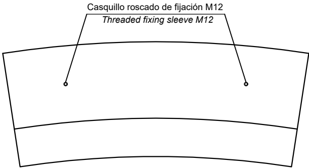
PLANTA INFERIOR / BOTTOM VIEW
