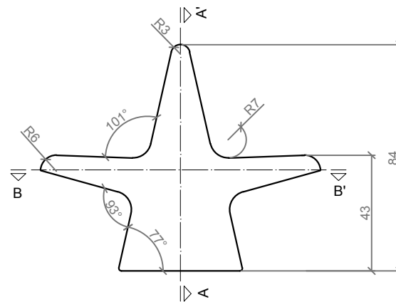
PERFIL / PROFILE
