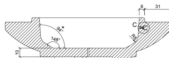
SECCION A-A' / SECTION A-A'
