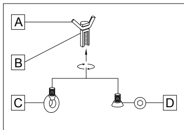
SISTEMA DE ELEVACION / LIFTING SYSTEM
